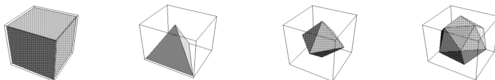
Figure 5A. Terre, feu, air et eau selon le modèle grec
