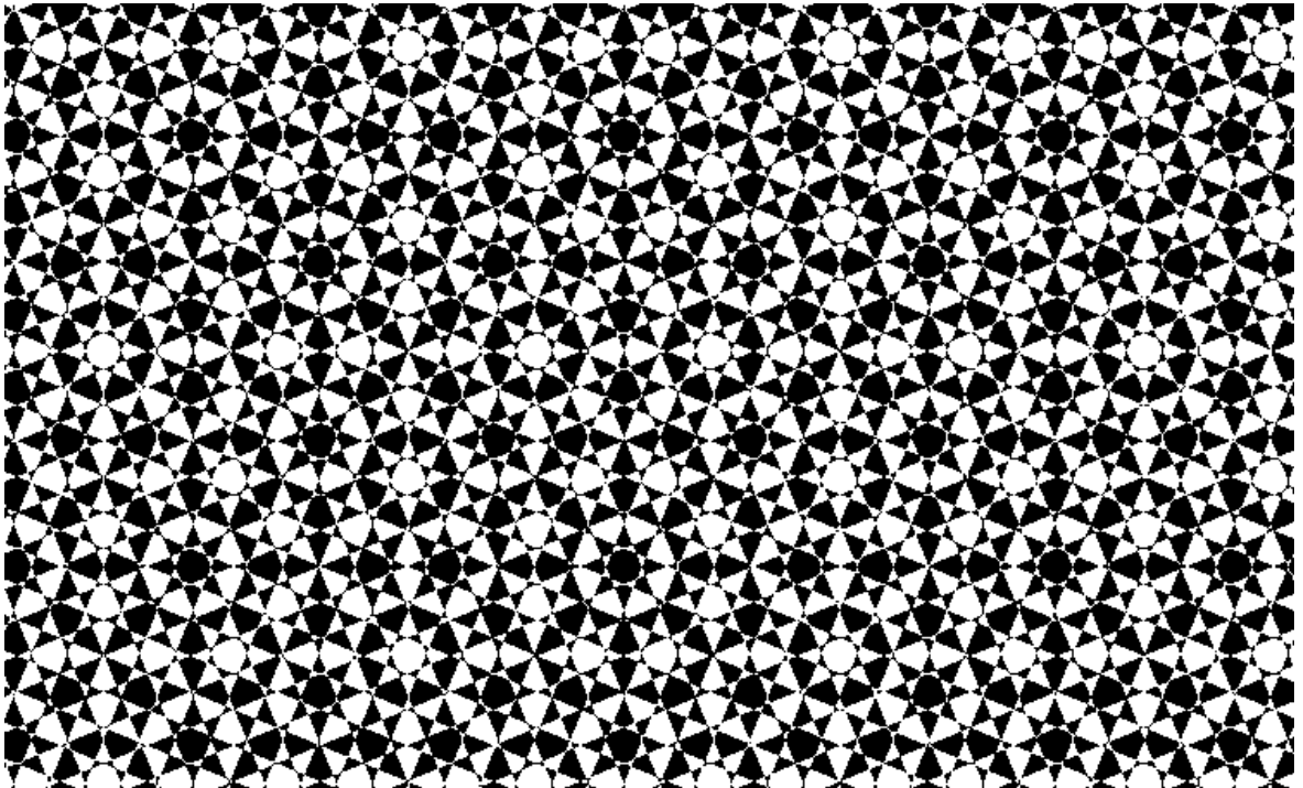
Figure 10 bis. Quasi – régularité
