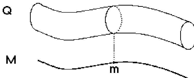
Figure 34. Une chose toute simple
