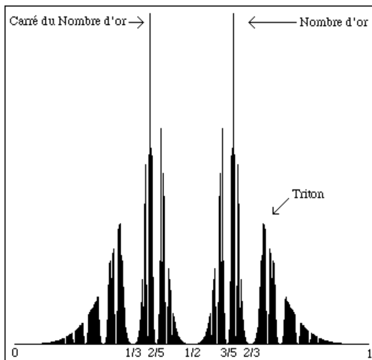
Figure 21. Échelle des dissonances
