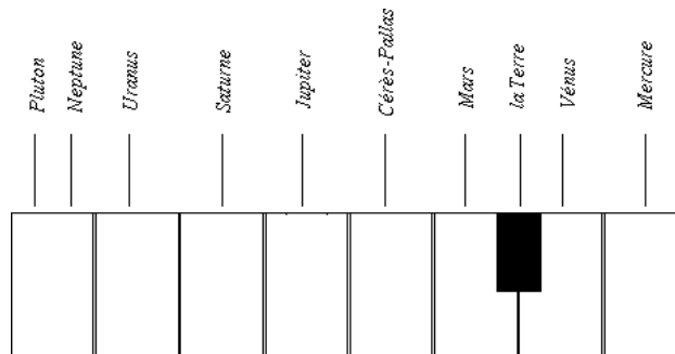
Figure 25. Gamme céleste achevée
