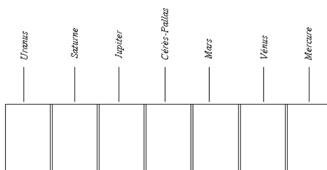
Figure 19. La gamme des planètes.
