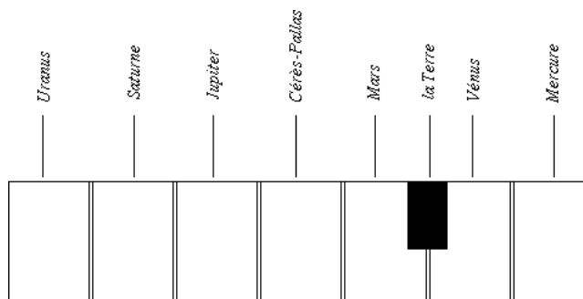
Figure 20. La Terre, en demi-ton...
