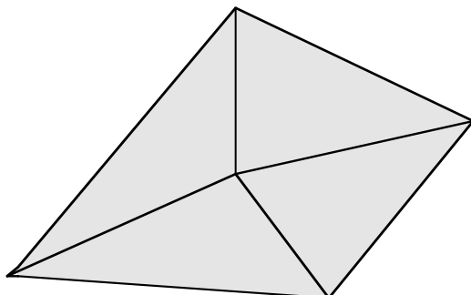
Figure 37 : les états purs, et les autres
