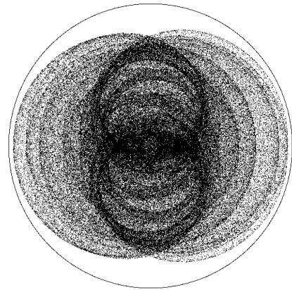
Figure 23. Apparition d'une régularité secrète
