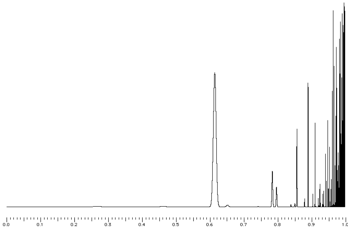
Figure 39. Spectre des fréquences des quatre planètes
