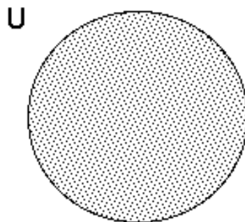
Figure 28 : simple portrait de l'Univers
