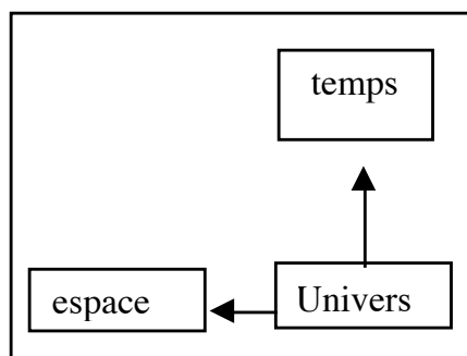
Figure 13. Pouvons-nous découper l'Univers ?
