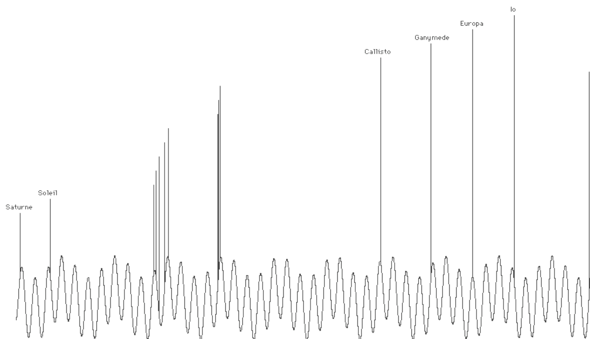
Figure 41. Dans le ciel de Jupiter
