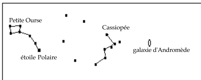
Figure 26. Pour les soirs d'automne
