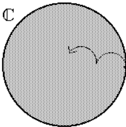
Figure 35. L'écran du hasard
