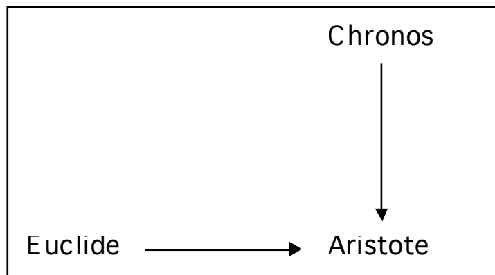
Figure 12. Voilà le groupe d'Aristote
