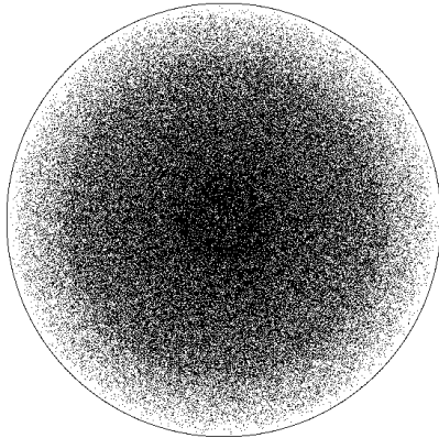
Figure 22. Des marées sur le Soleil
