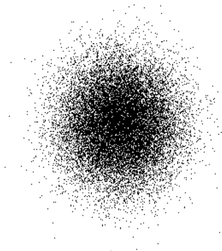
Figure 18. Un mouvement flou
