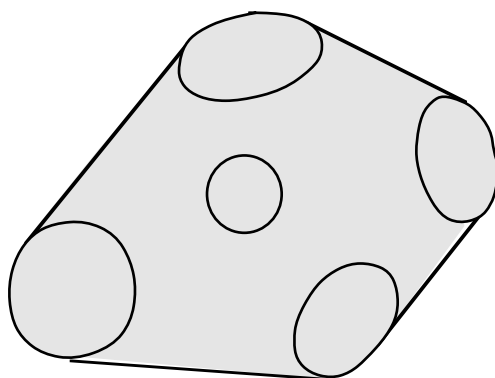
Figure 38 : ... donc elles sont ! "
