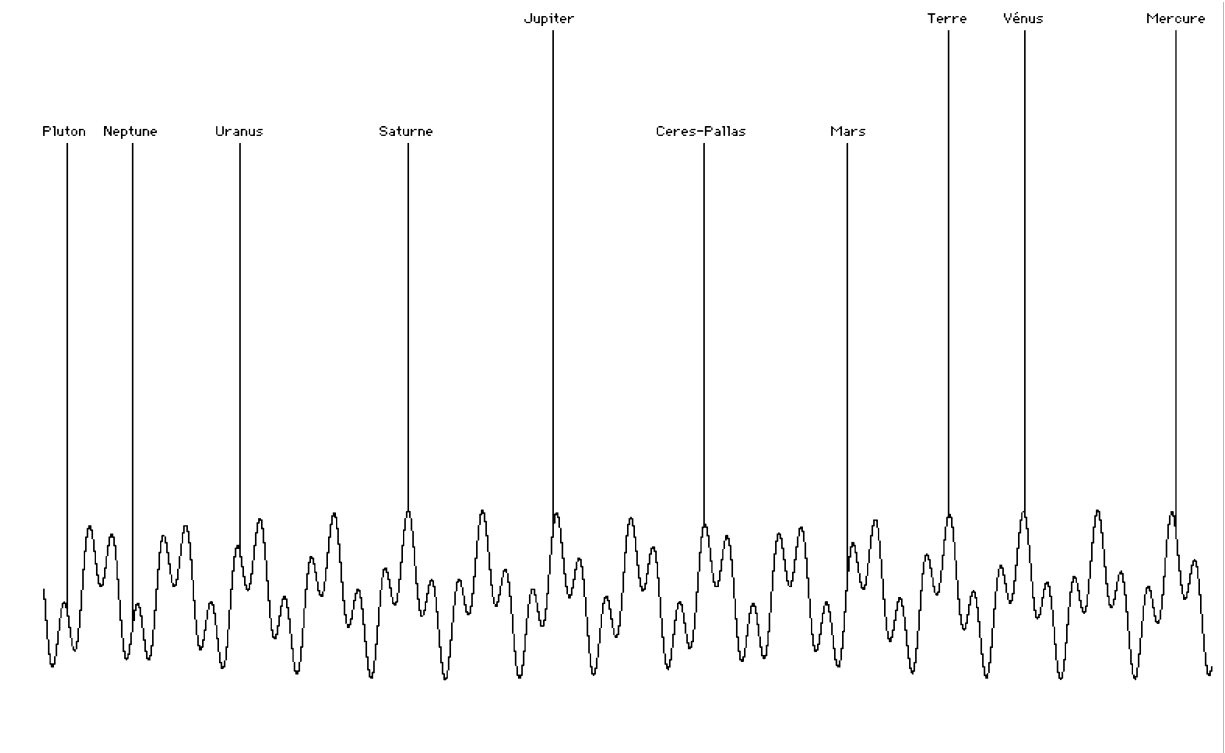
Figure 40. Apparition du système solaire
