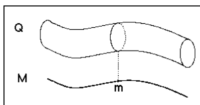
Figure 36: une chose parmi d'autres...
