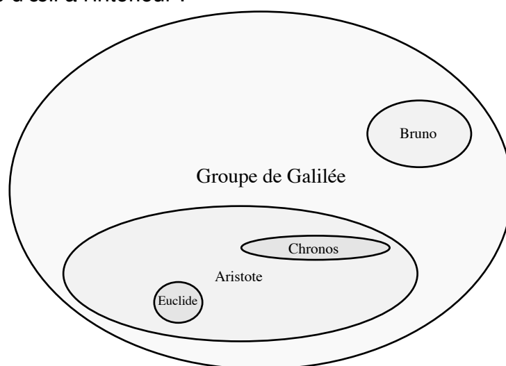
Figure 15 : Groupe de Galilée
