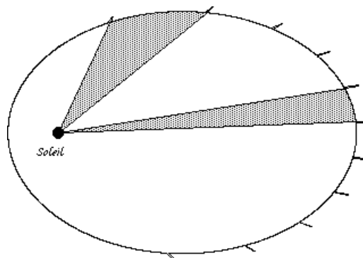
Figure 16. Course d'un astre
