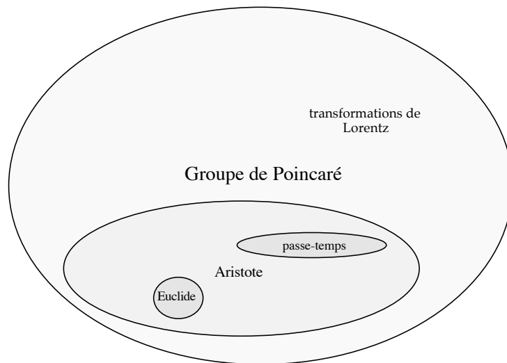
Figure 17. Groupe de Poincaré (3)
