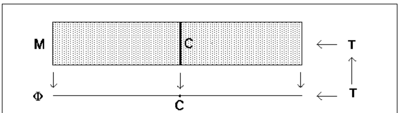
Figure 29 : types de métriques...
